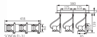
SONDA EL-3J
