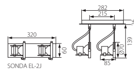
SONDA EL-2J
