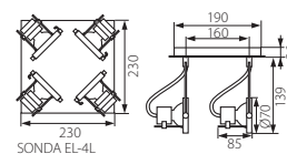
SONDA EL-4L
