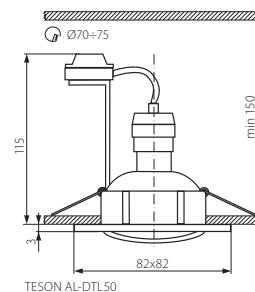
TESON AL-DTL50
