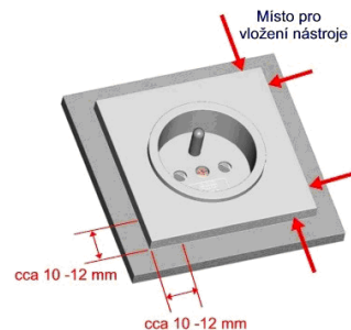
Obr. 11: Demontáž zásuvky Neo®
