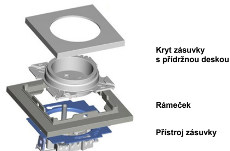
Obr. 10: Sestavování zásuvky Neo® s krytem a rámečkem
