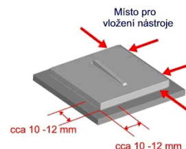
Obr. 9: Demontáž spínače Neo®
